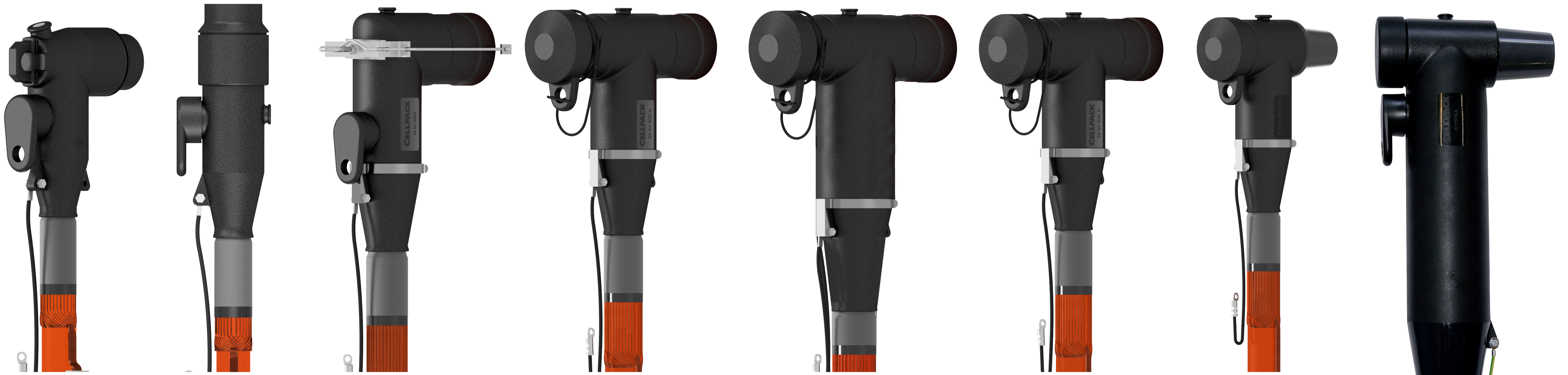
CWS 250A CGS 250A CWS 400A CTS 630A CTS 1250A CTS-S 630A CTKS 630A CTKSA acodado recto acodado en T asimétricos en T simétrico de acople pararrayos
