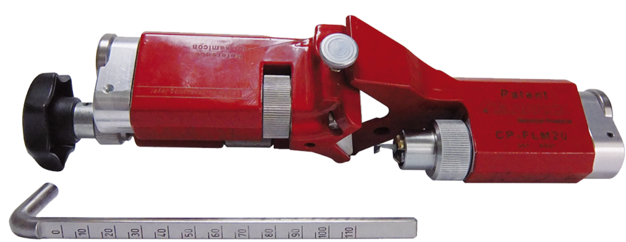
FLM20 | peladora de cubierta aislamiento y semiconductor
