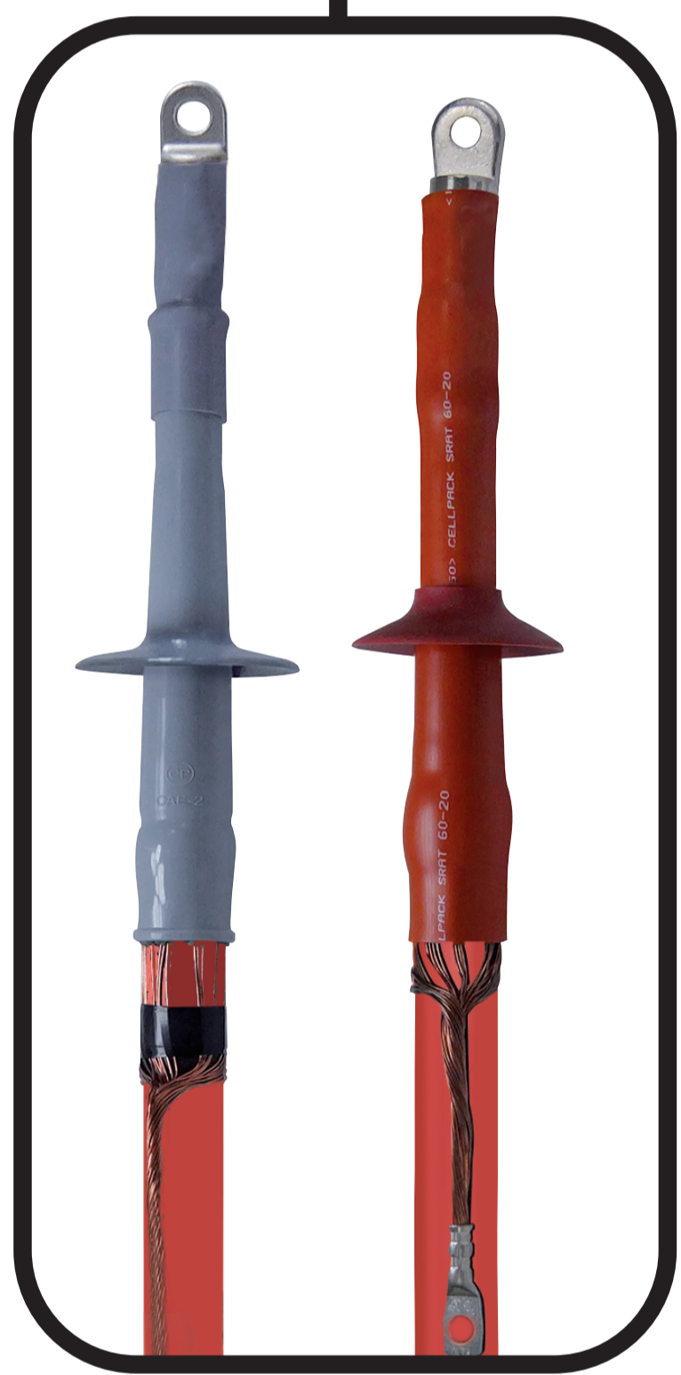
CAESK-I/CHESK-I Terminación de interior
